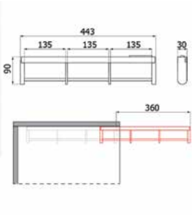
Porte-vêtements coulissant T.443 - charge: 10 kg
